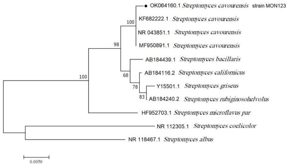
شکل ۹- درخت تبارزایی که با نرم‌افزار MEGA 7 با روش پیوست همسایه‌ها (Neighbor-joining) براساس تبادف قسمتی از ژن 16S rRNA در جدایی (MON123) جدا شده از Satureja khuzestanica و جدایی‌هایی از ژن بانک با بوت‌استرپ ۱۰۰۰ تکرار رسم شده است. استرین جدا شده در این مطالعه با دایره سیاه در کنار آن در درخت تبارزایی مشخص شده است و شماره‌های دسترسی مربوط به آن‌ها نوشته شده‌اند. گونه‌ی Streptomyces albus به عنوان گروه خارجی انتخاب شد
